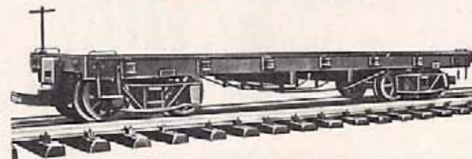
4060 Plattformwagen, LüP 380 mm 4achsrig, braun, mit Rungen, Pinzgauer Lokalbahn und US-Bahnen DM 24,50
