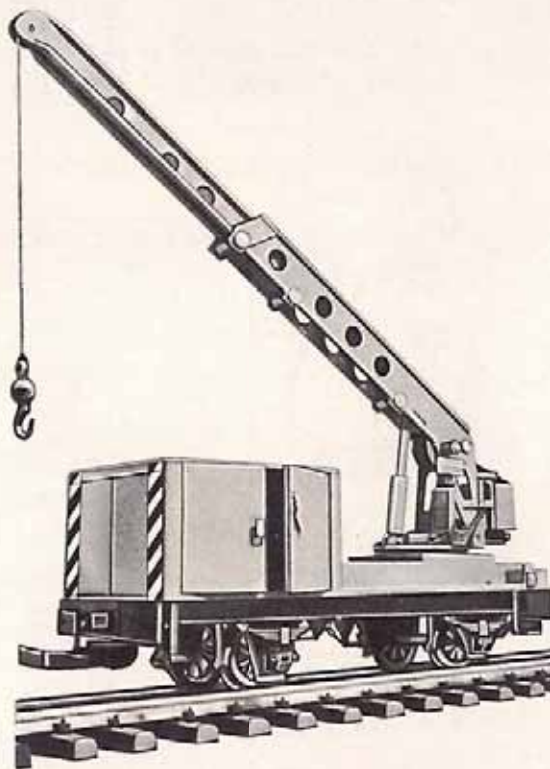
4042 Kranwagen, LüP 300 mm gelb, Typ MATRA DM 42,50
